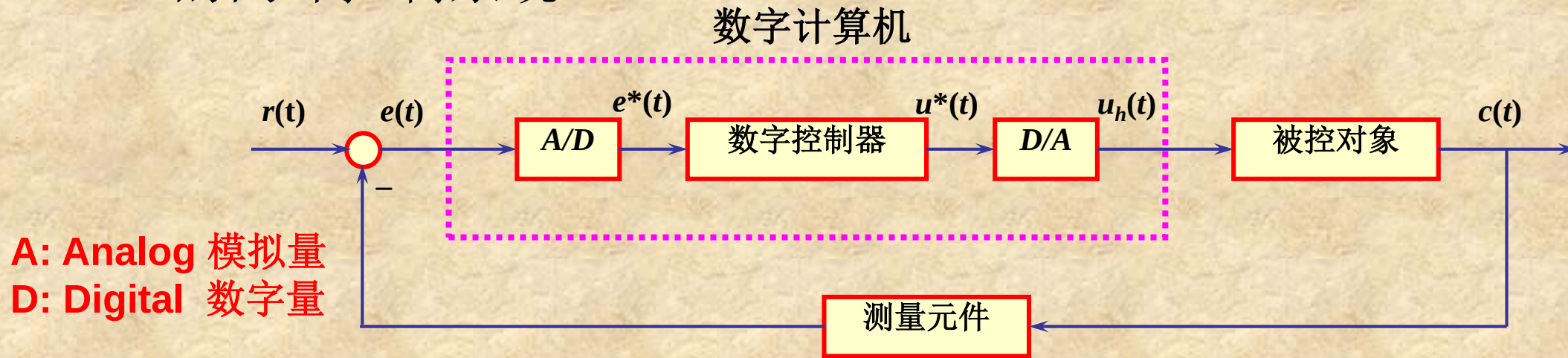
计算机控制系统典型原理图
