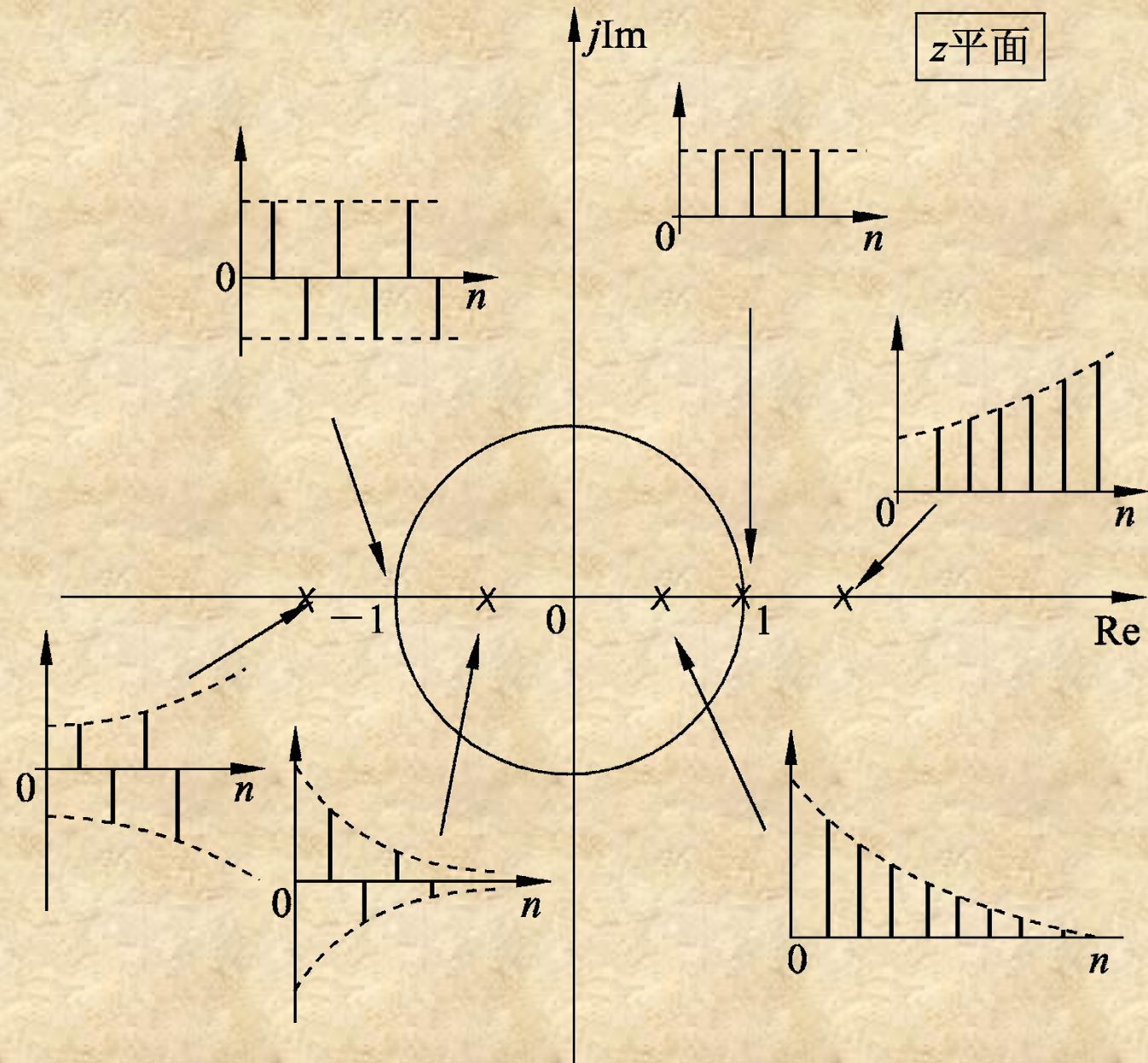
闭环实极点分布与相应的动态响应形式
