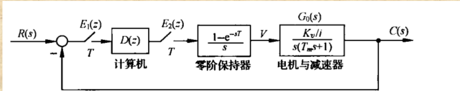
图 7-46 有纹波最少拍系统
